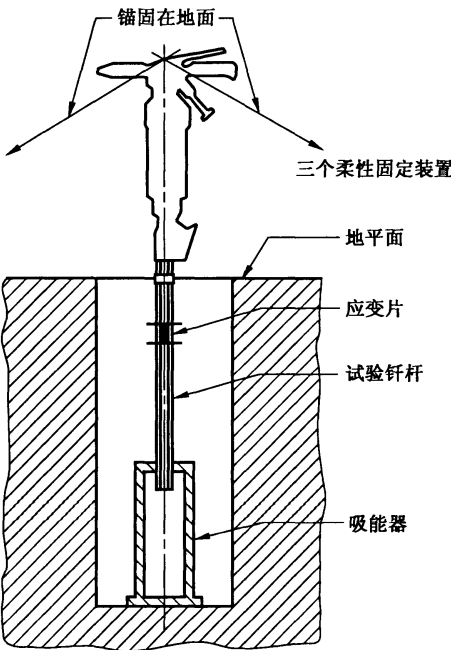
图 C.1 应变测量装置
